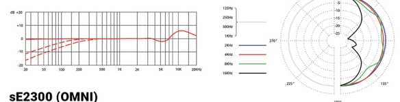
sE2300 (OMNI)
